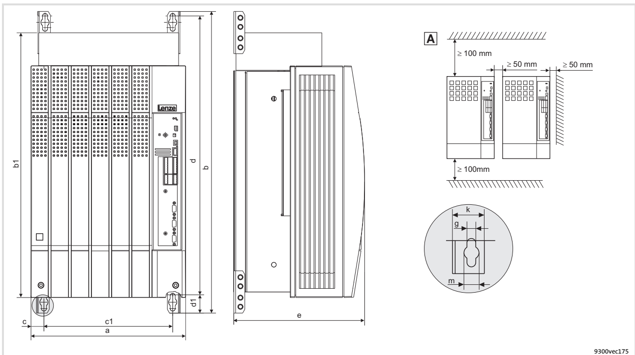
Abb. 4-9 Standardmontage mit Befestigungswinkeln 55 kW
