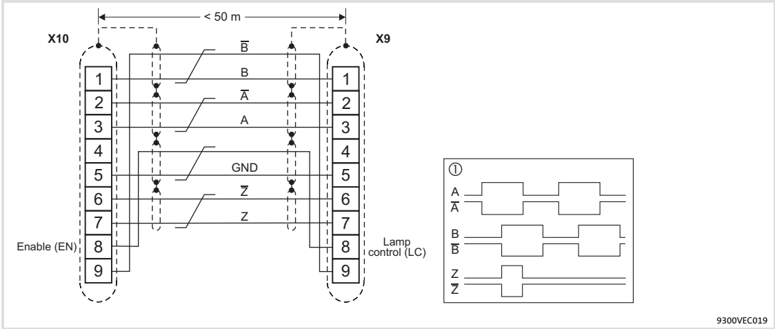
Abb. 5-17 Anschluss Leitfrequenzeingang (X9) / Leitfrequenzausgang (X10) X9 Folgeantrieb (Slave) X10 Leitantrieb (Master) ① Signale bei Rechtslauf / Paarweise verdrehte Adern
