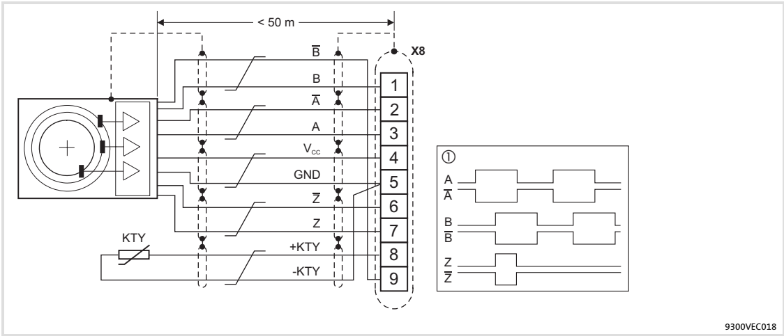
Fig.5-15 Raccordement du codeur incrémental avec niveau TTL (RS-422) ① Evolution des signaux en cas de rotation horaire / Brins torsadés par paire
