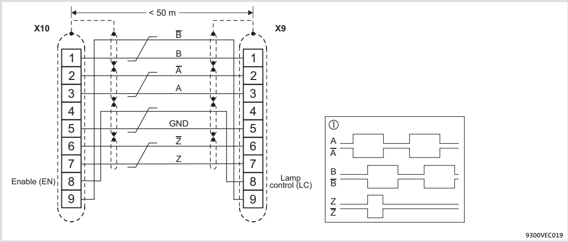
Fig.5-23 Raccordement de l'entrée fréquence maître (X9)/de la sortie fréquence maître (X10) X9 Entraînement esclave X10 Entraînement maître ① Evolution des signaux en cas de rotation horaire Brins torsadés par paire
