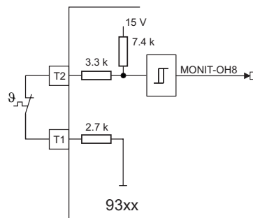
Eingangsschaltung für T1, T2
