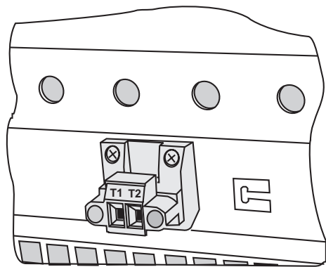
Klemmen T1, T2 am Antriebsregler
