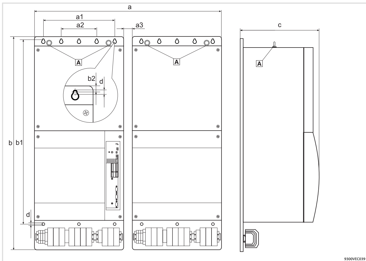
Fig.3-1 Encombrements [A] Anneaux de levage
